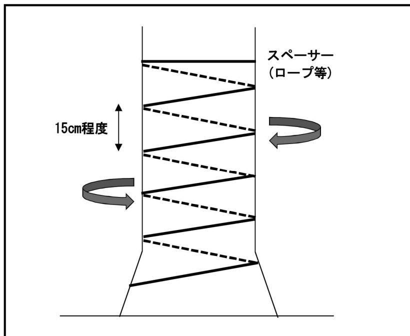
図4 スペーサーの設置方法
