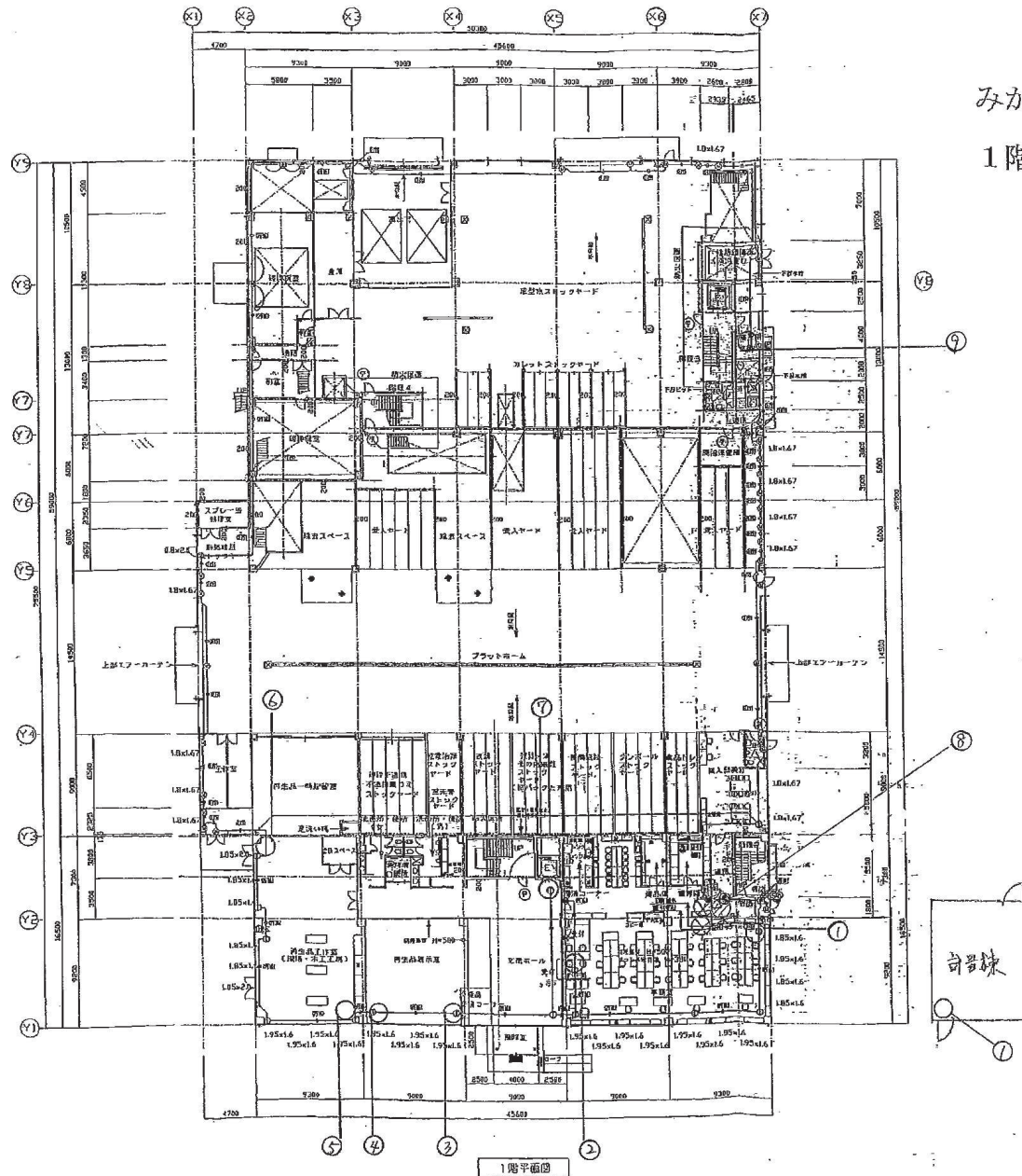
1階平面図
