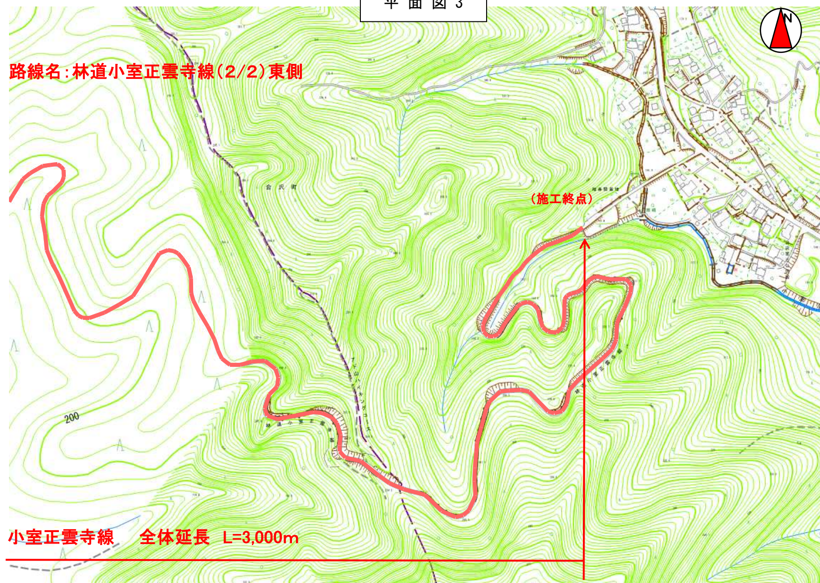
平面図 3
