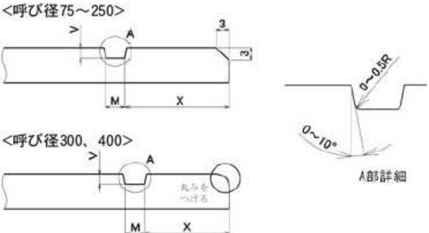
図 2-4 GX形ダクトイル鋳鉄管の挿し口加工寸法
