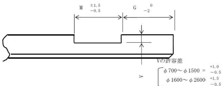
図 2-3 UF、UF-D形ダクト用鋳鉄管の挿し口加工寸法
