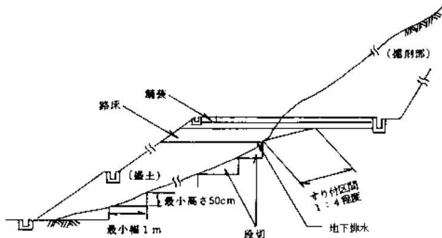
図 4-2 盛土基礎地盤の段切り
