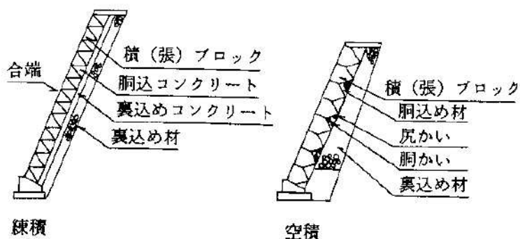
図 3-3 コンクリートブロック工
