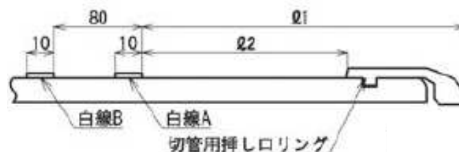
図 2-5 GX形ダクタイル鋳鉄管の白線表示位置
