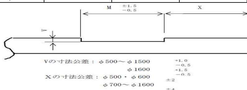
図 2-2 S形ダクトイル鋳鉄管の挿し口加工寸法
