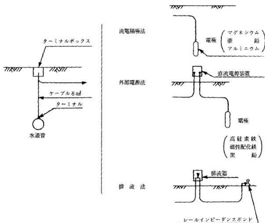
図 2-9 防食装置参考図
