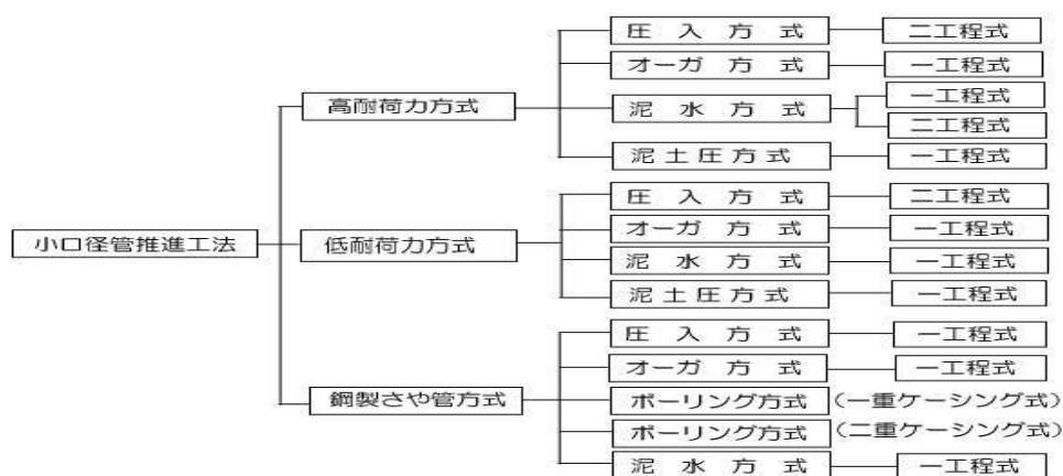
図 2-10 小口径管推進工法の分類
