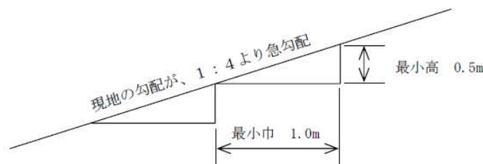
図 4-1 盛土基礎地盤の段切り
