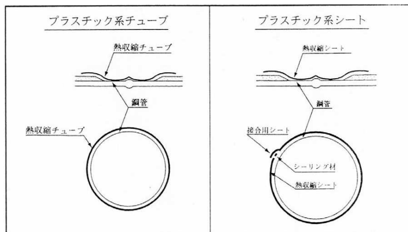
図 2-7 ジョイントコートの巻付け
