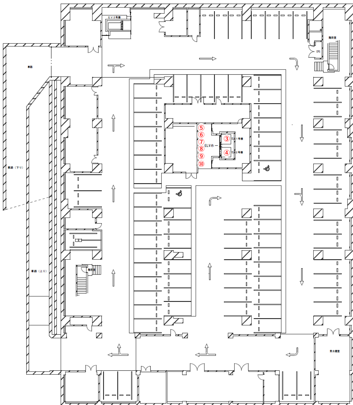
地下平面図
