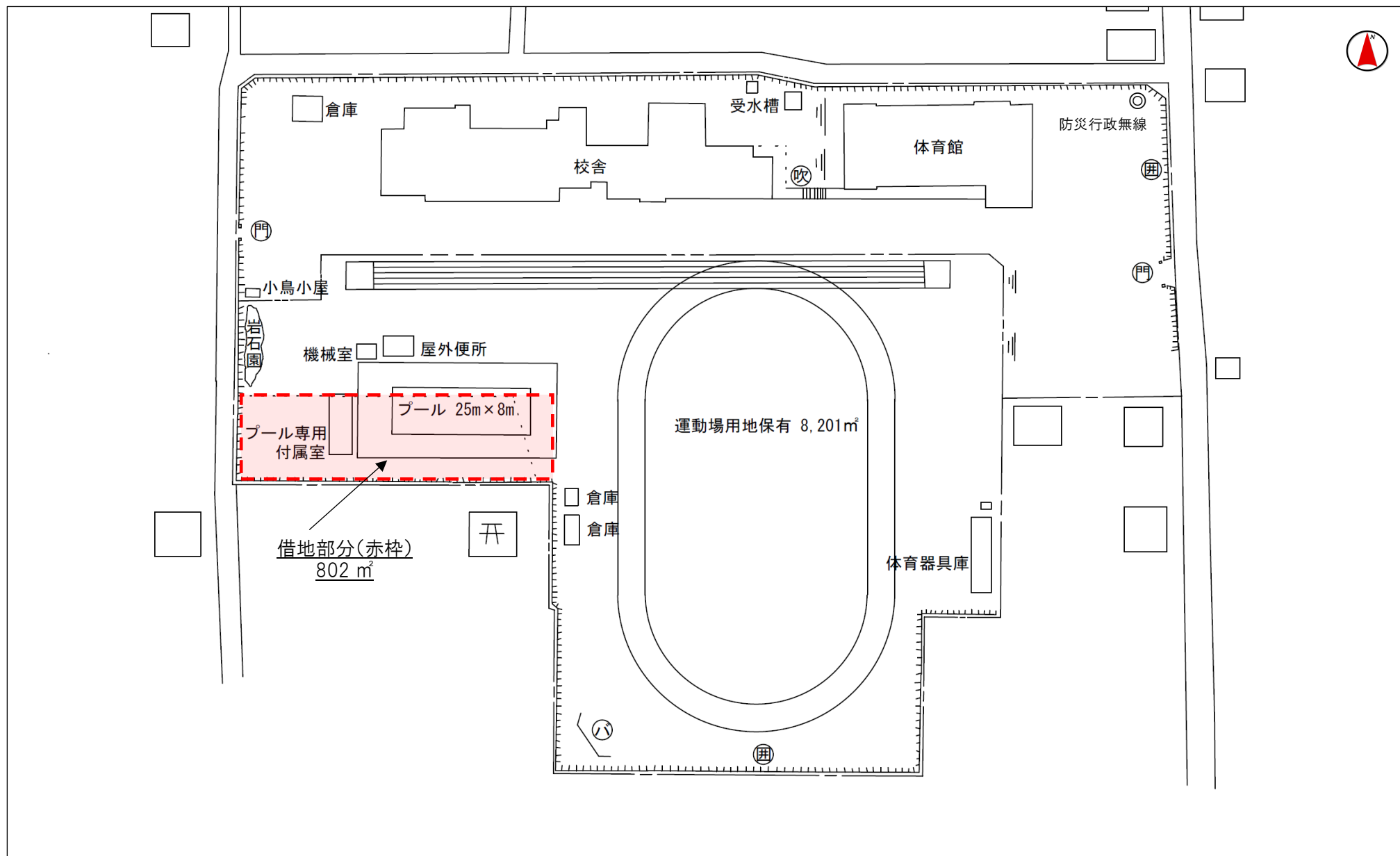
旧飛駒小学校 配置図
