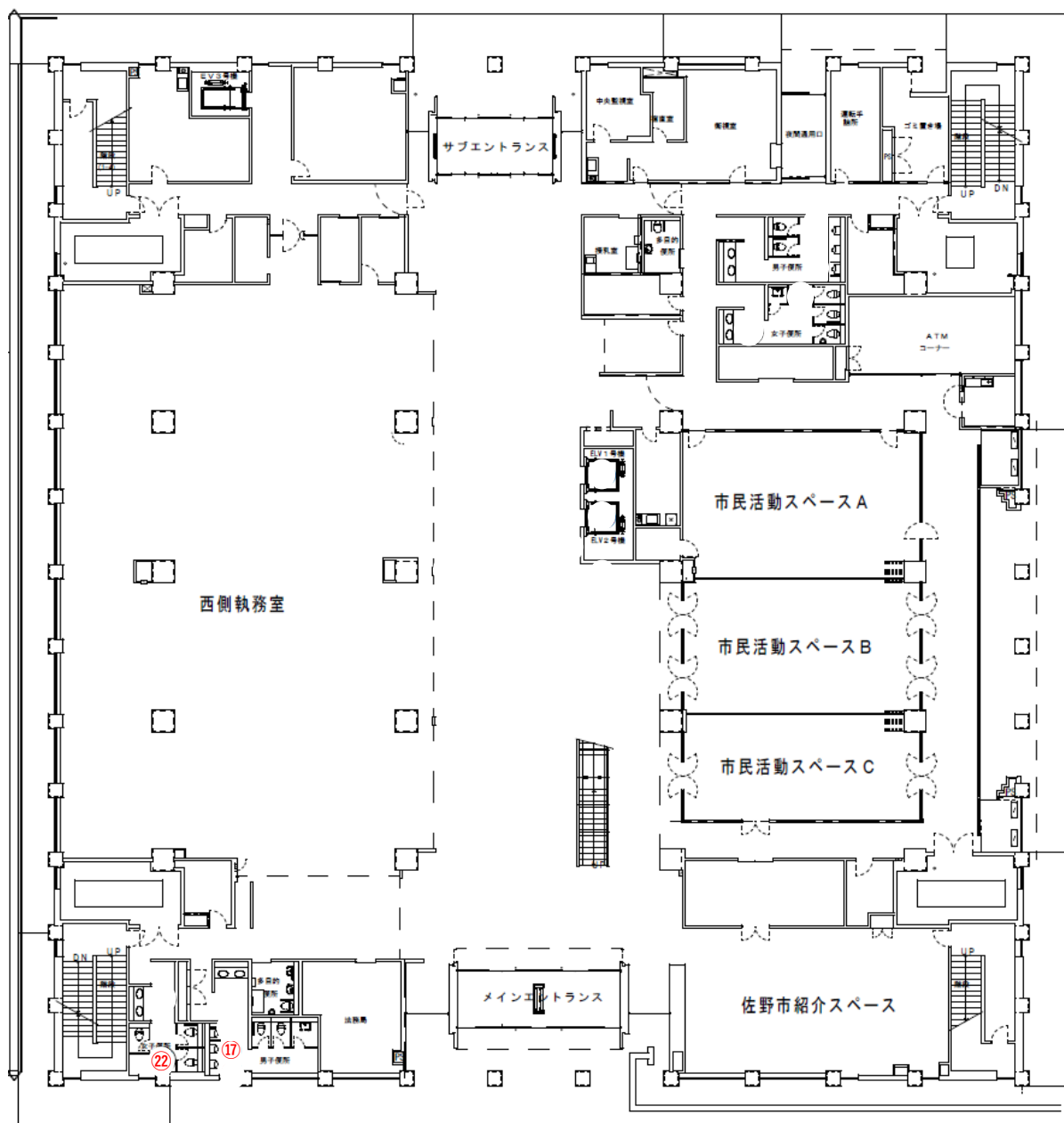
1 階平面図
