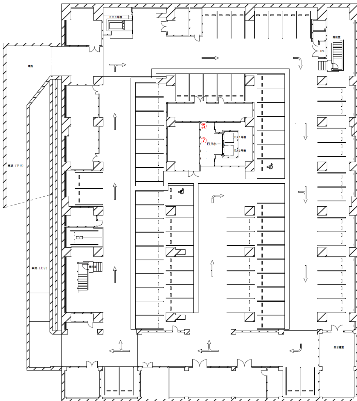
地下平面図
