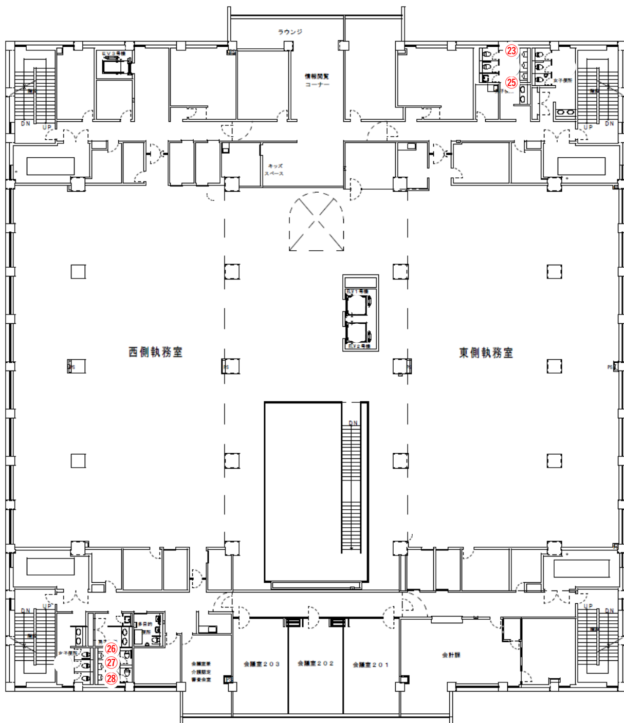
2 階平面図
