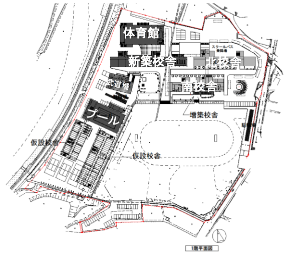
計画図
