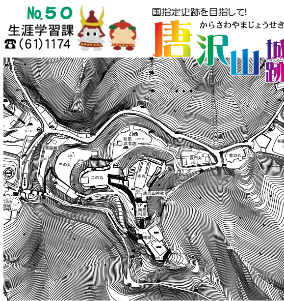
第11図 山頂主要部測量図
