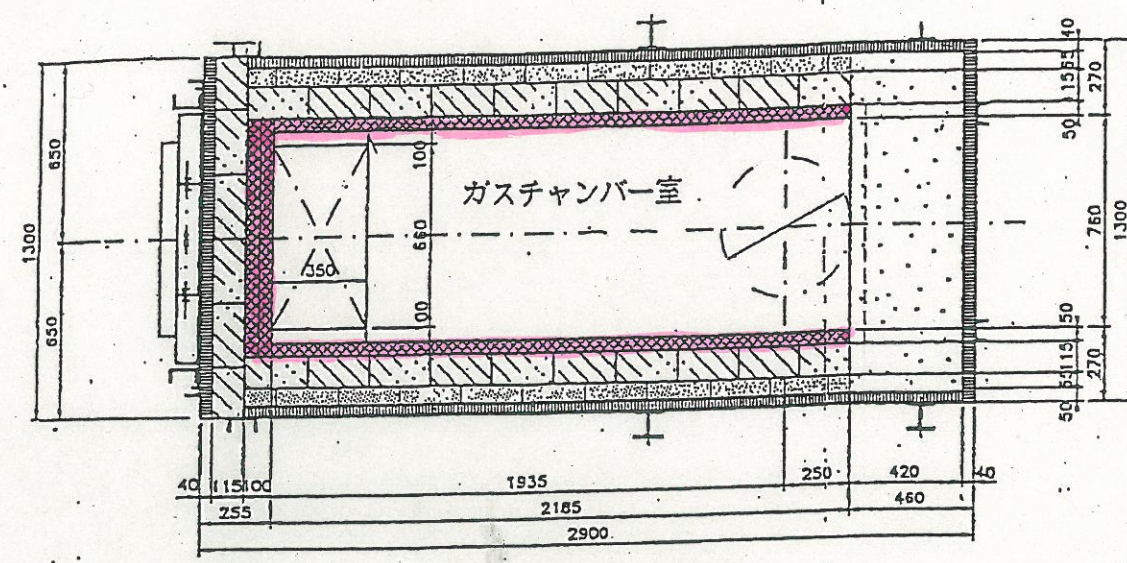
B-B 断面図
