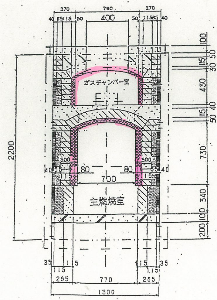
E-E 断面図
