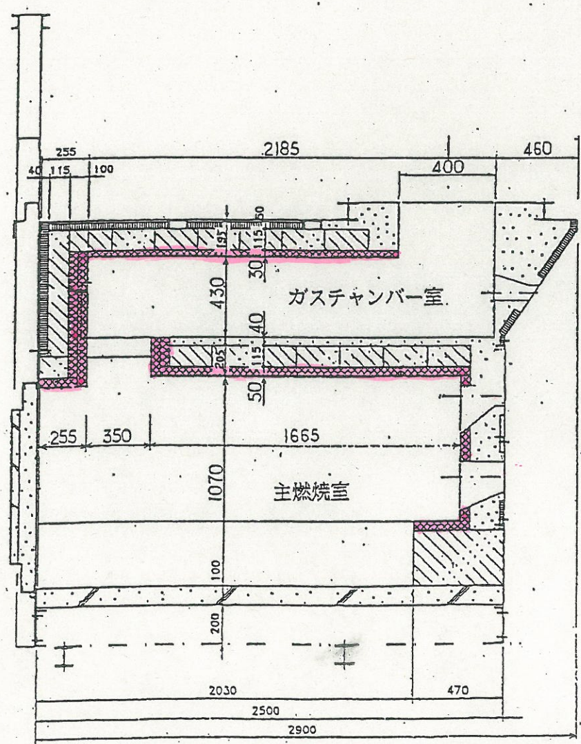
C-C 断面図
