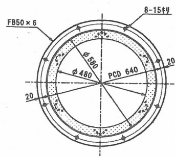
②下段排気筒
