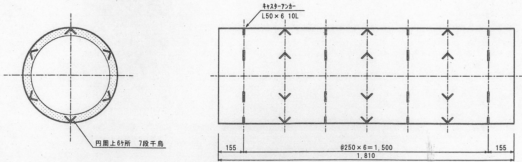
③キャスターアンカー（上、下段排気筒）
